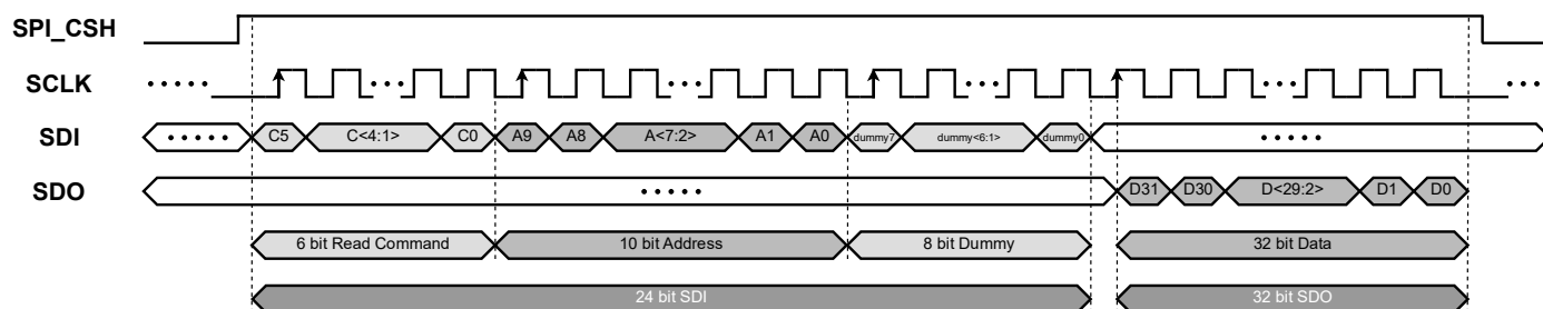
图 7-2. SPI 读数据接口波形
