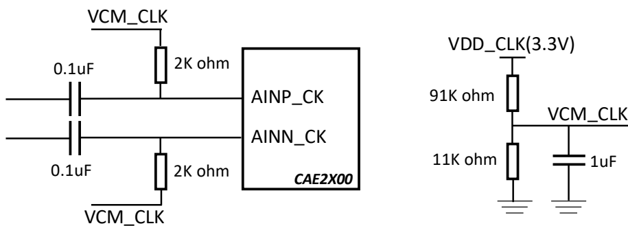
图 8-4. 主时钟输入管脚交流 (AC) 耦合连接示意图
