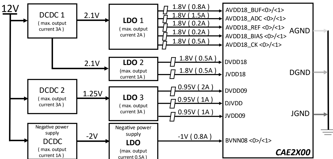
图 8-12. CAE2200 推荐电源连接示意图
