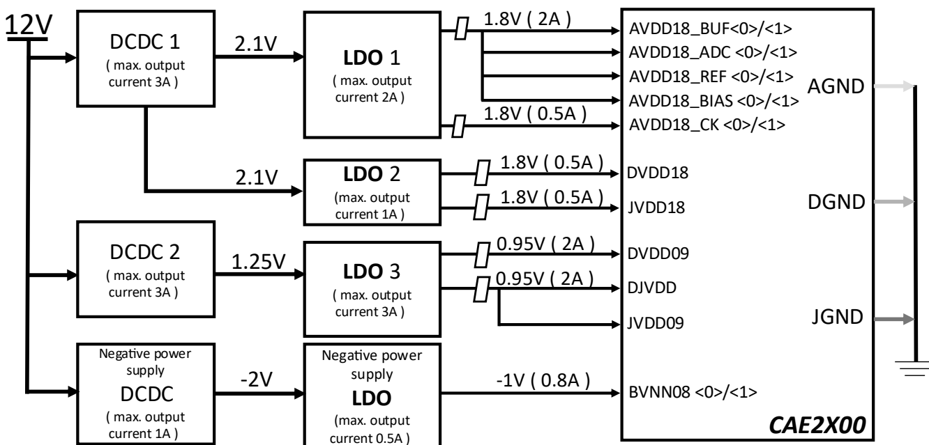
图 8-13. CAE2200 推荐合并电源连接示意图
