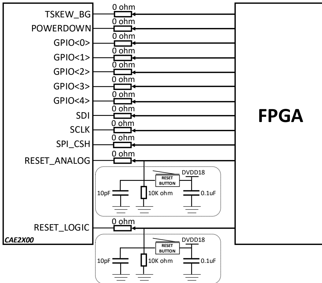
图 8-9. 数字 IO 输入管脚 (1.8V 电平) 连接示意图
