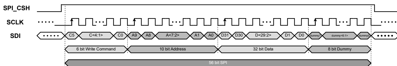
图 7-1. SPI 写数据接口波形
