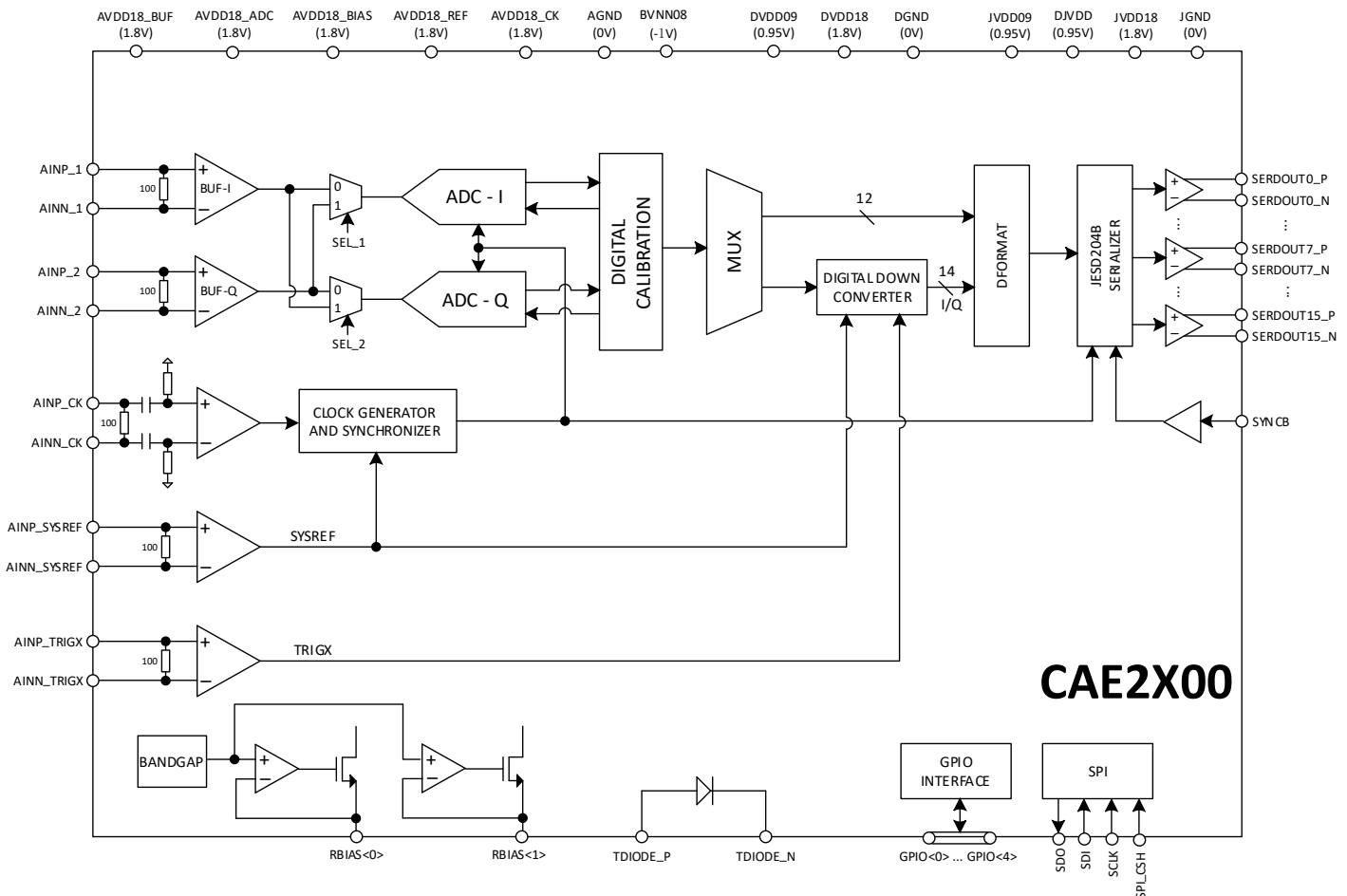
图 8-1. 功能框图
